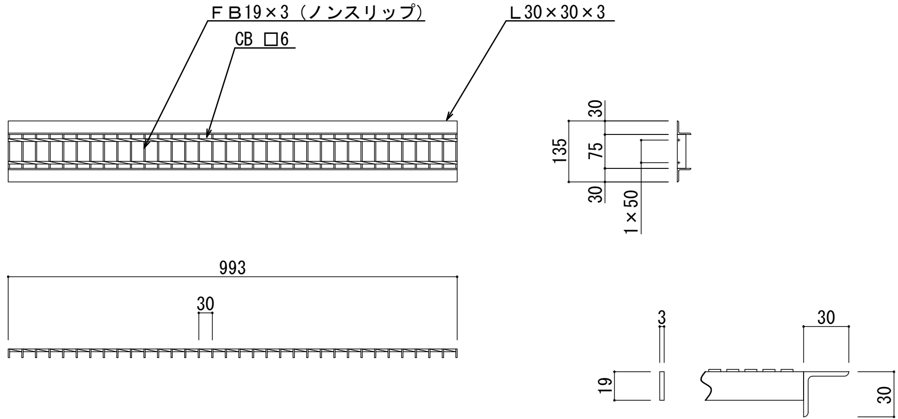
断面詳細
