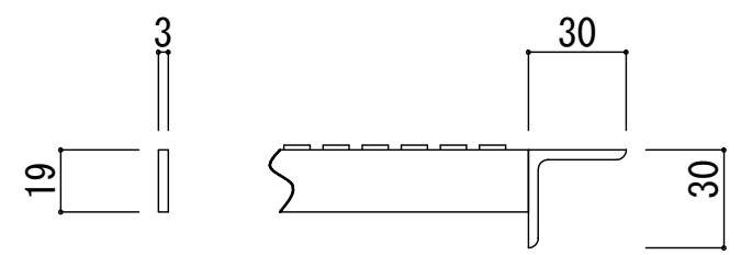
断面詳細
