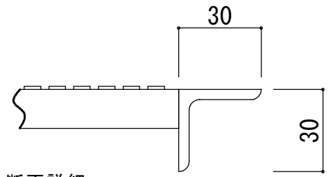
断面詳細
