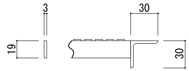
断面詳細
