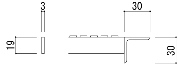
断面詳細
