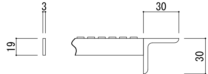
断面詳細
