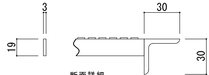
断面詳細
