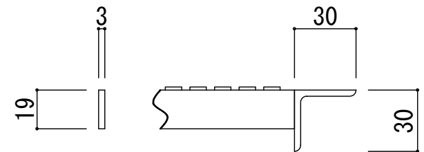
断面詳細
