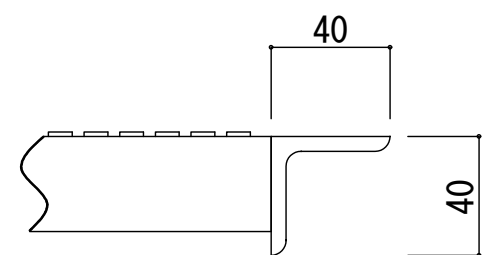
断面詳細図
