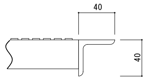
断面詳細図
